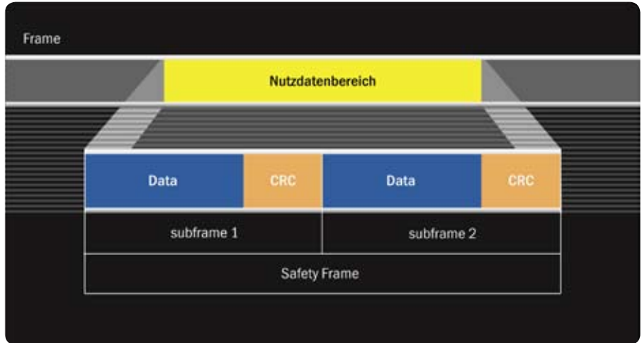
Der SAFETY Frame wird im Nutzdatenbereich eines Standardframes transportiert. Er besteht aus zwei identischen Subframes, die jeweils mit einer eigenen Prüfsumme gesichert werden.
