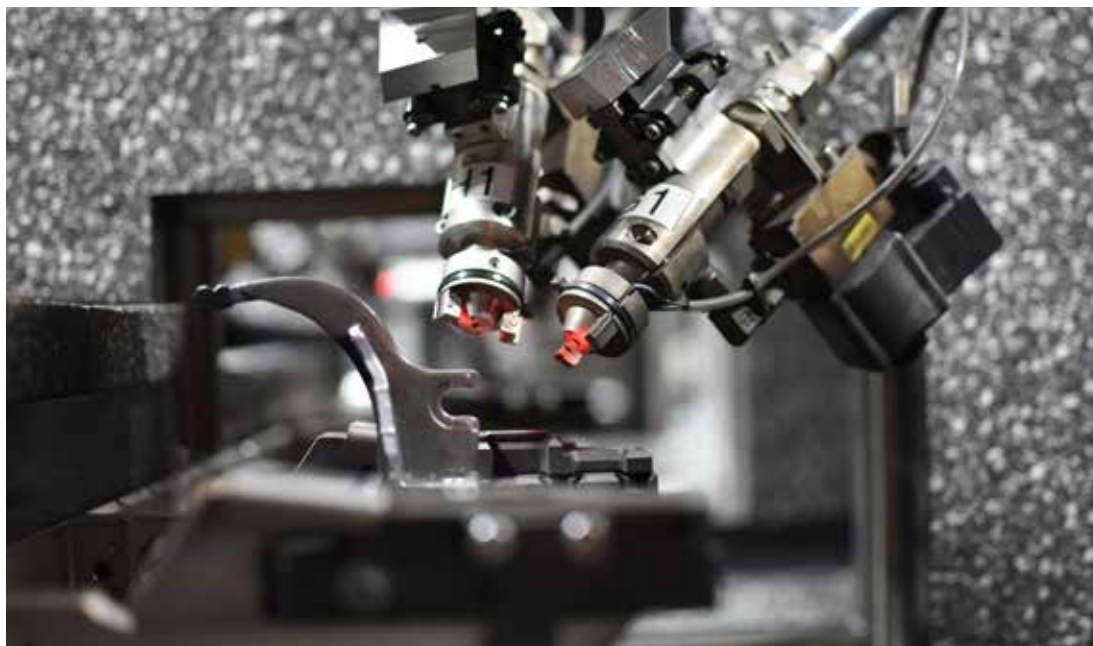
Eine bis fünf fest montierte JetModul-Düseneinheiten pro Reinigungskammer bearbeiten die bis zu 20 Schweißnähte der Laserschweißbaugruppen.
